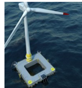
OCEAGEN – IDEOL
