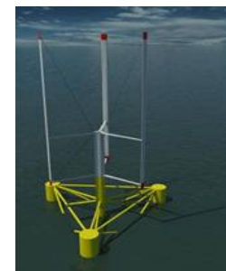
VERTIWIND - TECHNIP
